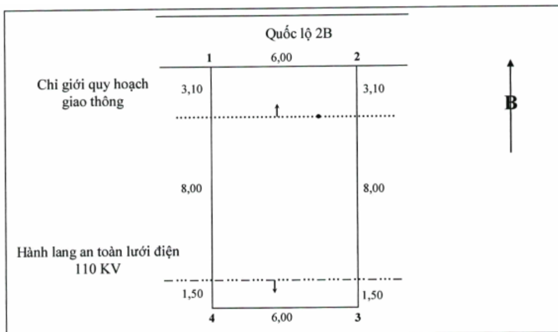
Hình 2. Sơ đồ thửa đất có nhiều cạnh thừa
